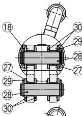
View A-A
