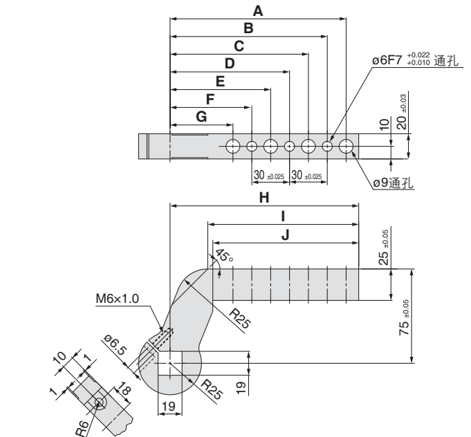
50mm偏置型—有加工孔
