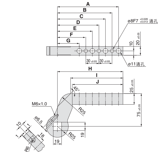
50mm偏置型—有加工孔
