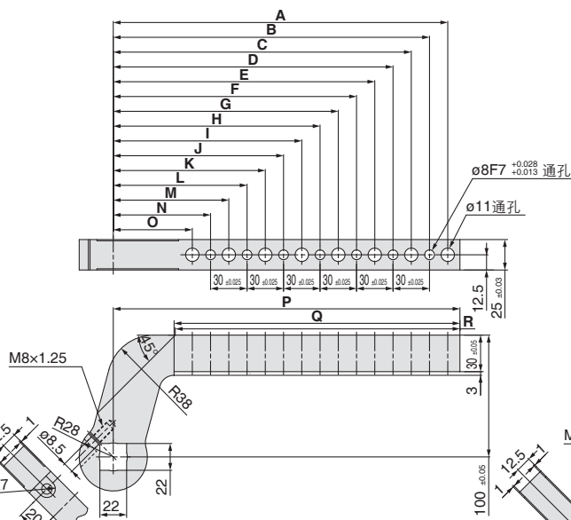
70mm偏置型-有加工孔
