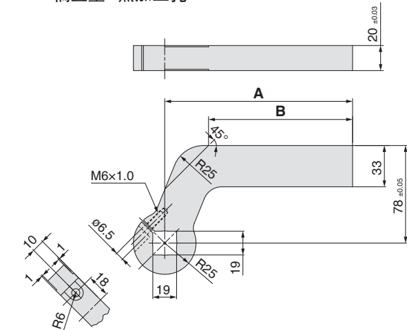
45mm偏置型—無加工孔
