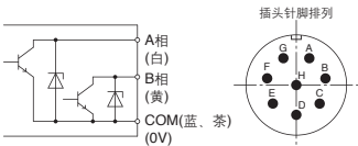
行程可读气缸的输出回路
