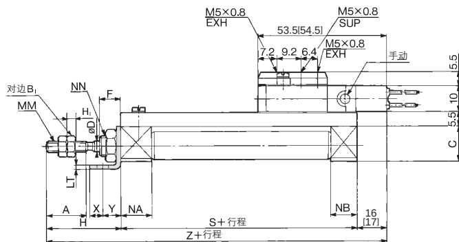
杆端螺母
