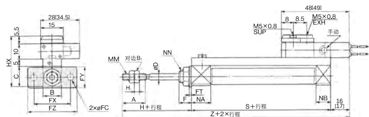
杆端螺母
