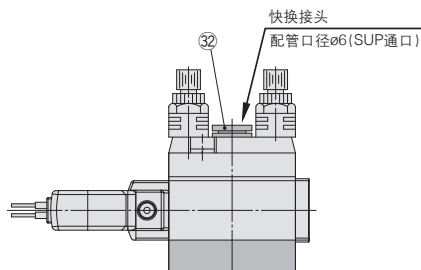
内置快换接头的场合
