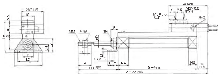
杆端螺母
