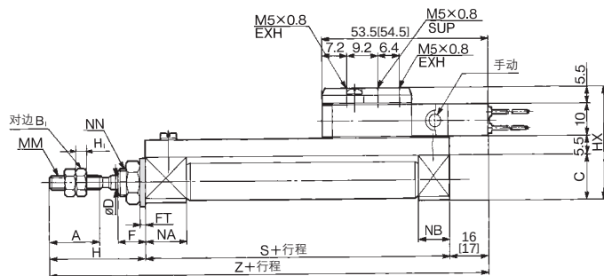
杆端螺母
