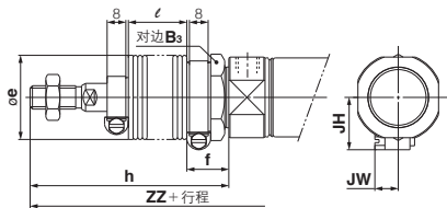
带防护套
