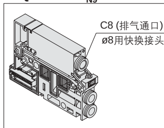
单独排气用隔板 VVQ2000-R-1-C8 N9
