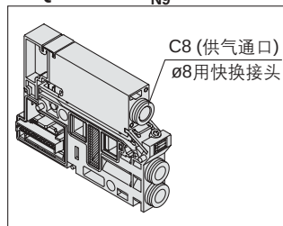
单独供气用隔板 VVQ2000-P-1-C8 N9
