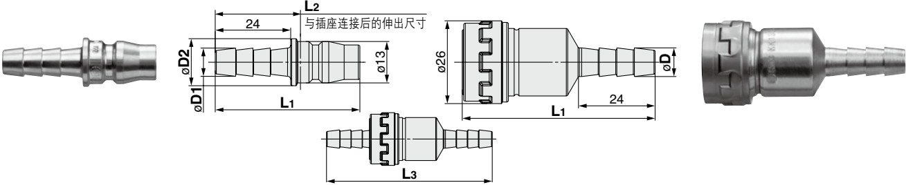
倒钩接头型(适用橡胶管)
