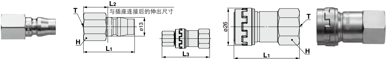
内螺纹型
