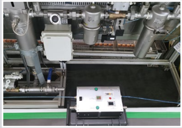
设备管路泄漏检测：可检测1L/min以上的泄漏
