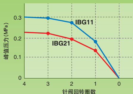
峰值压力和针阀回转圈数 (供给压力: 0.5MPa)
