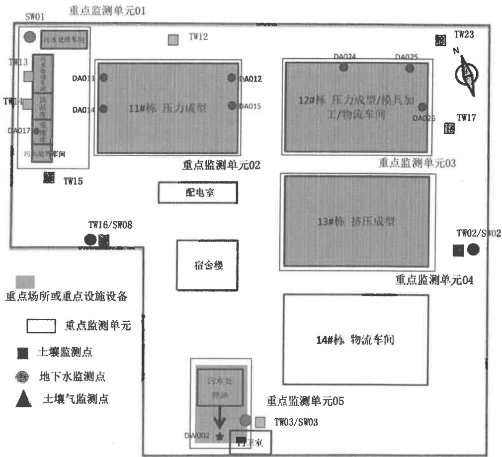
图 6-1 监测点位布设（北厂）
