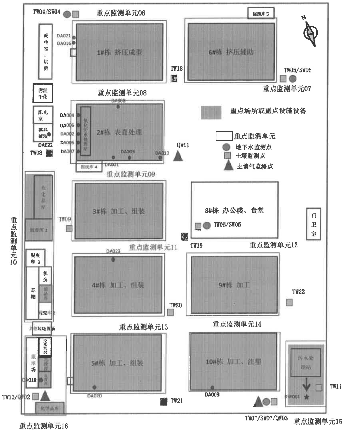
图 6-2 监测点位布设 (南厂)
