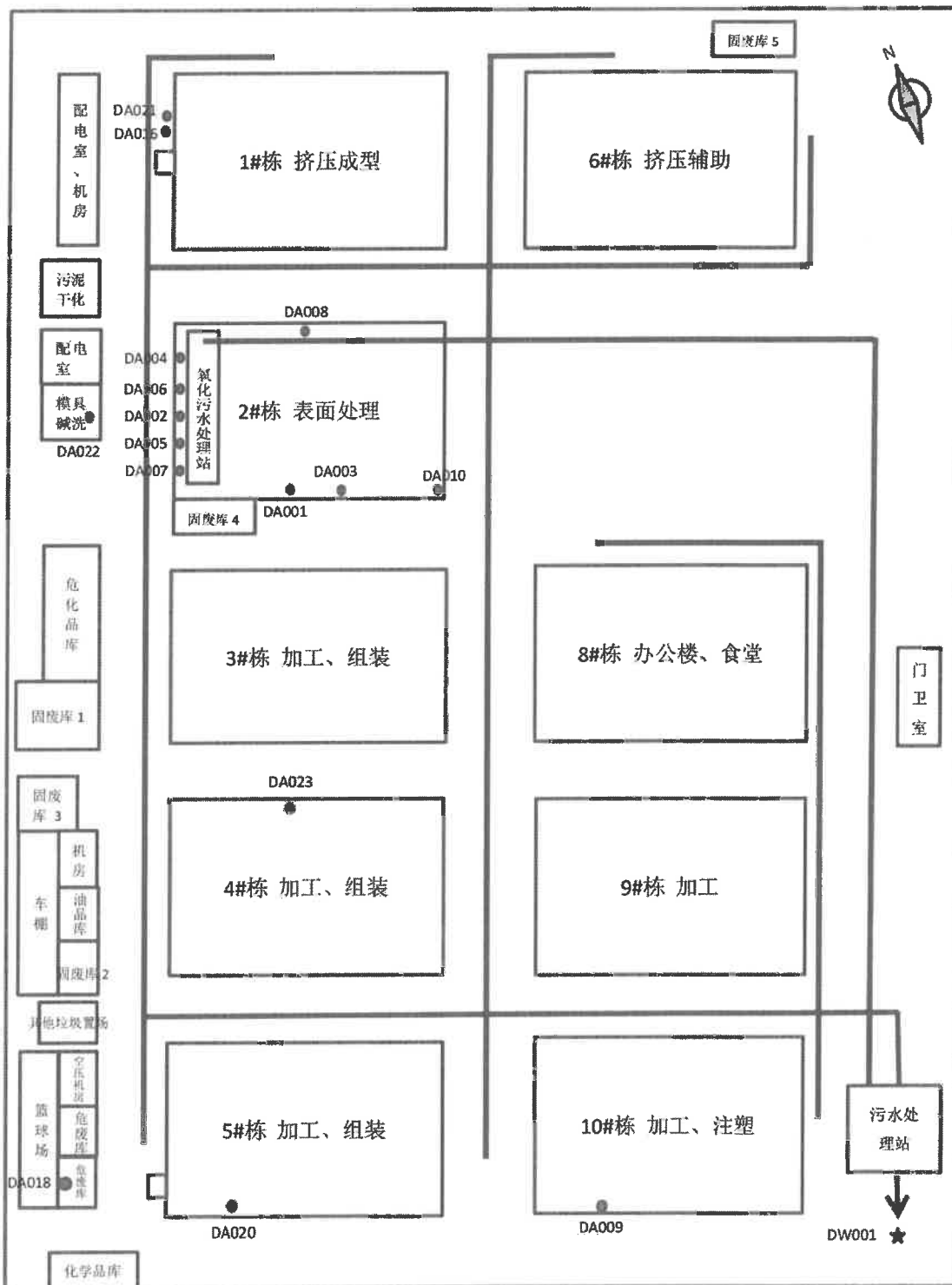
图 4-3 南厂平面布置图
