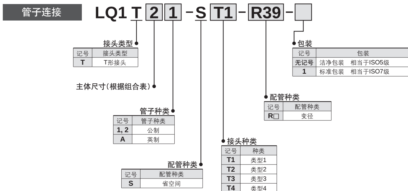
组合表(公制)
