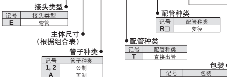
组合表(英制)
