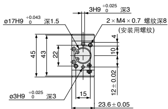
磁性开关安装用槽位置
