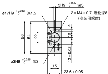
磁性开关安装用槽位置
