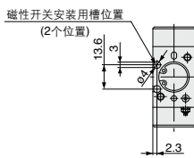
磁性开关安装用槽位置
