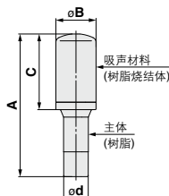
尺寸表 (mm)
