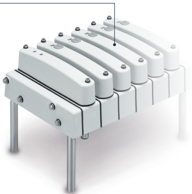
洁净型集装阀岛 导线型 JSY5000-H 系列
