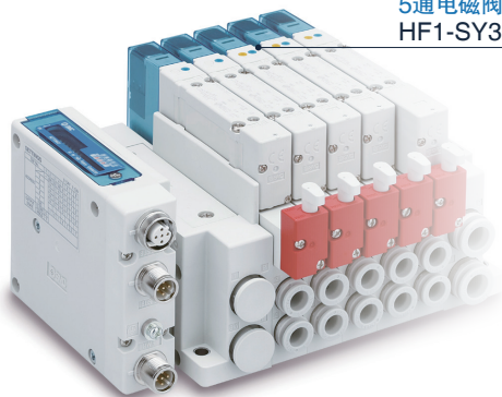
· 5通电磁阀 直接配管型 / 单体 HF1-SY3000/5000/7000 系列
