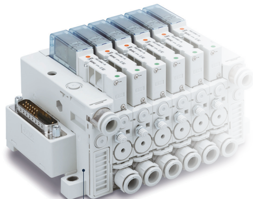
真空单元 HF1-ZK2□A 系列
