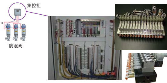
电气控制柜的定制与改造 —集装式电磁阀VFS2100系列
